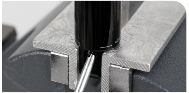
Schrader-Ventileinsatzwerkzeug
