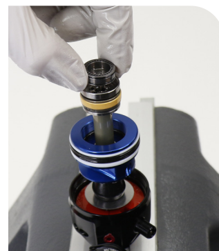
Kolbenwerkzeug / 14-mm-Stecknuss
