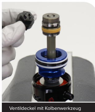
Ventildeckel mit Kolbenwerkzeug
