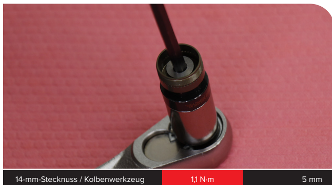
14-mm-Stecknuss / Kolbenwerkzeug
