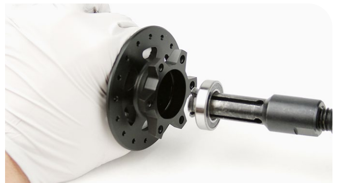
Geschlitzter 17-mm-Aufsatz
