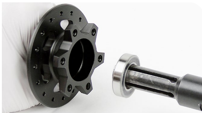
Geschlitzter 17-mm-Aufsatz
